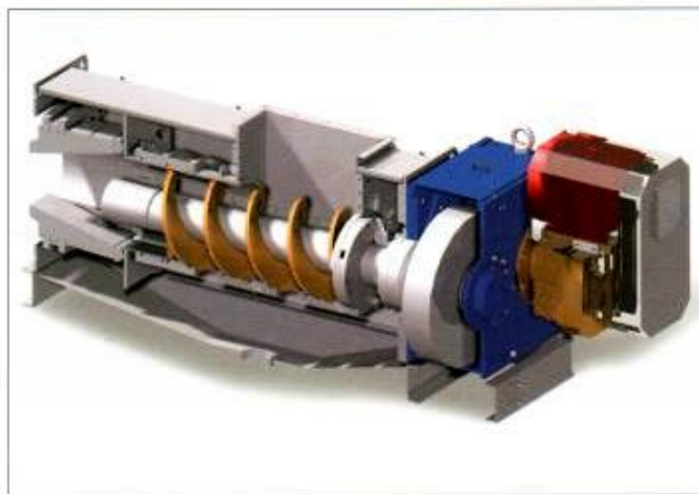
Die BP-Beltec Schneckenpresse erreicht Spitzenwerte im Trockengehalt
